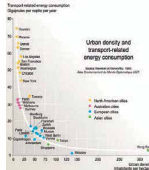
De grafiek 'Urban density and transport-related energy consumption' (Newman & Kenworthy), toont de relatie tussen dichtheid en het vervoers-gerelateerde energieverbruik.
